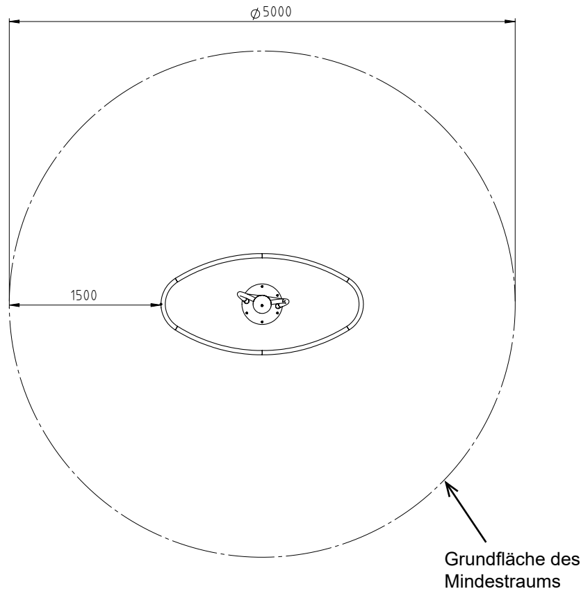
Skizze 3: Draufsicht
