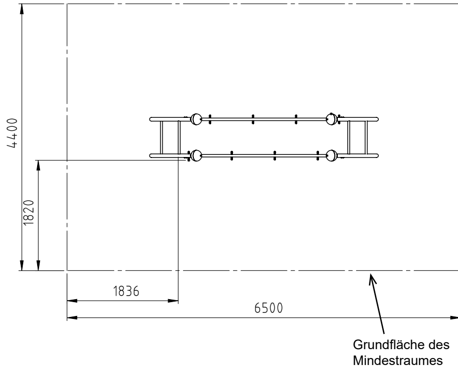
Skizze 3: Draufsicht
