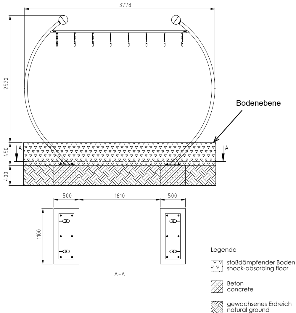
Skizze 2: Fundamentplan
