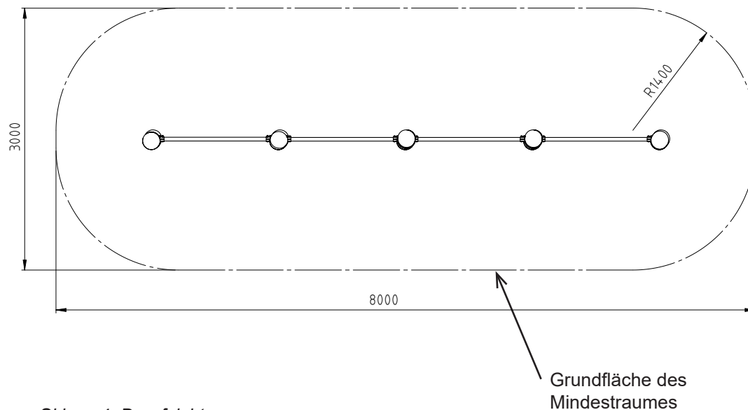
Skizze 4: Draufsicht
