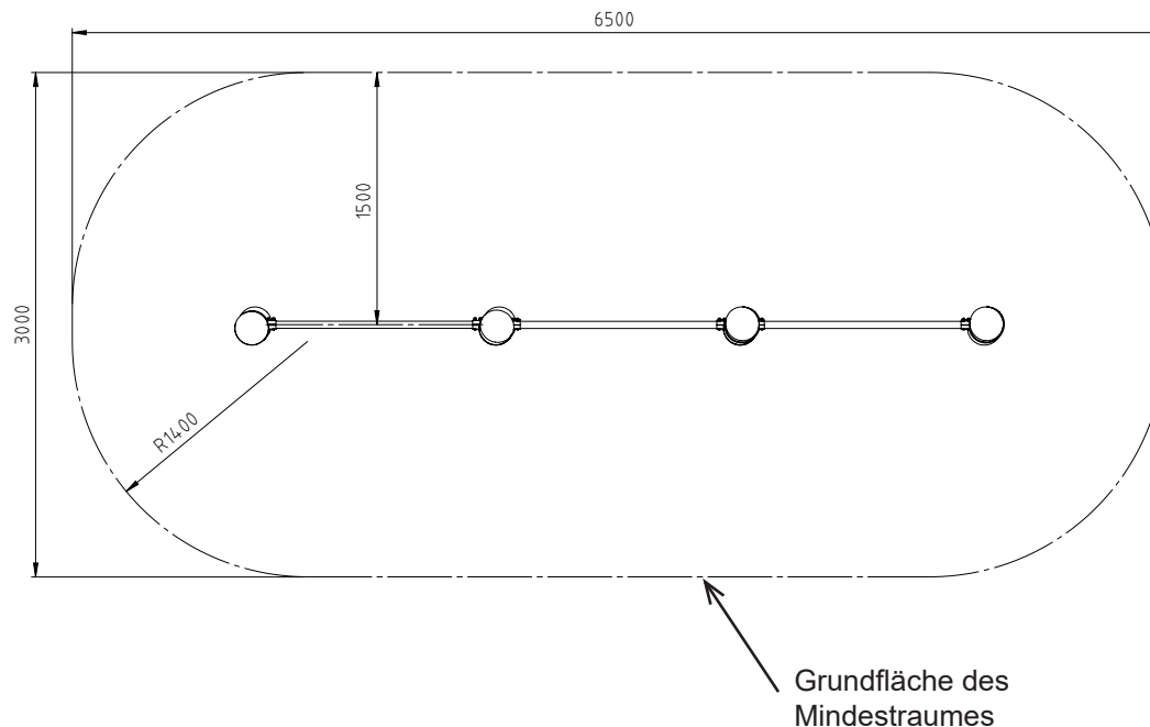
Skizze 4: Draufsicht
