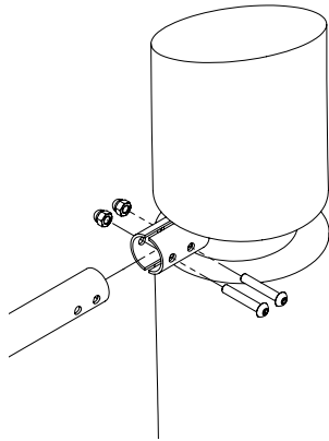
Skizze 3: Zusammenbau
