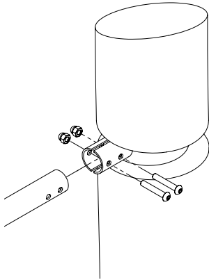
Skizze 3: Zusammenbau
