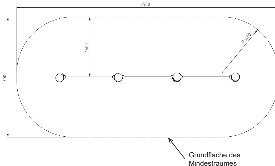
Skizze 4: Draufsicht
