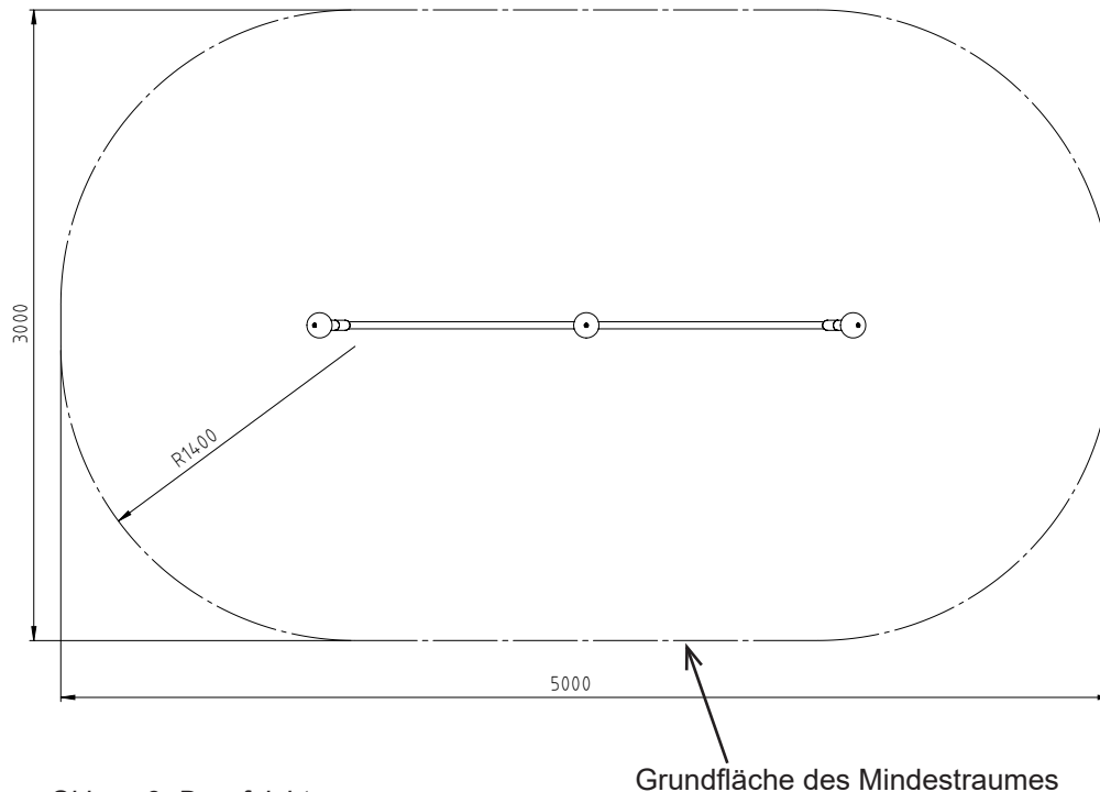
Skizze 3: Draufsicht
