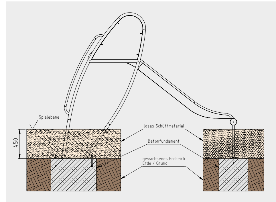
Fundamentüberdeckung mit losem Schüttmaterial Einbautiefe: 450 mm
