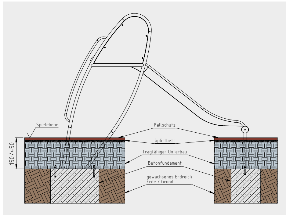
Fundamentüberdeckung mit synthetischem Fallschutz Einbautiefe: 150 mm oder 450 mm
