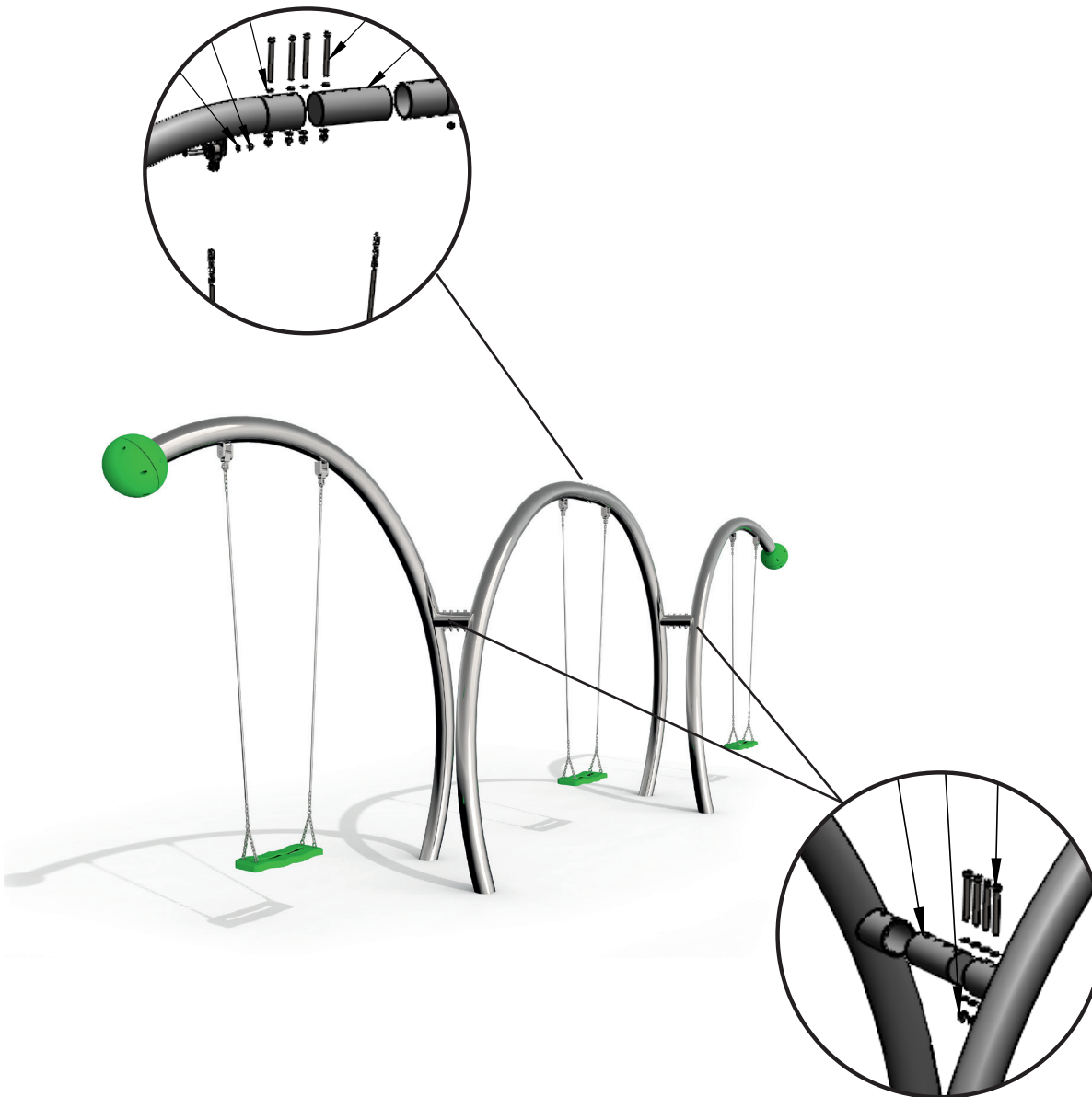
Skizze 3: Montage
