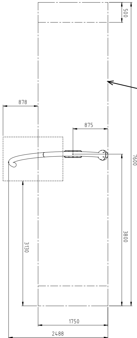
Skizze 3: Draufsicht
