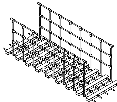
Skizze 4e: Anbauteil: „Wackelbrücke“
