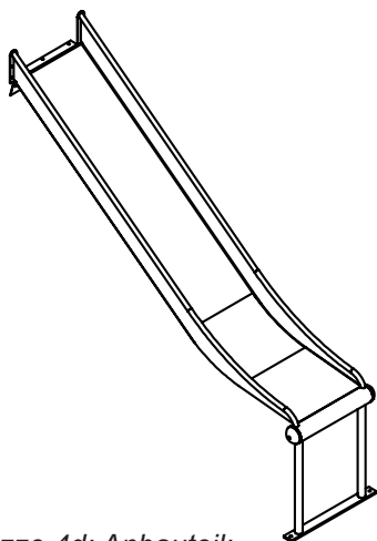
Skizze 4d: Anbauteil: „Rutsche“
