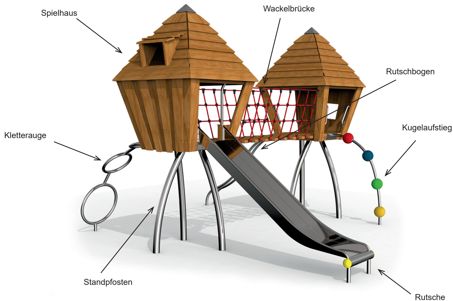
Skizze 1: Gesamtansicht des Spielgerätes
