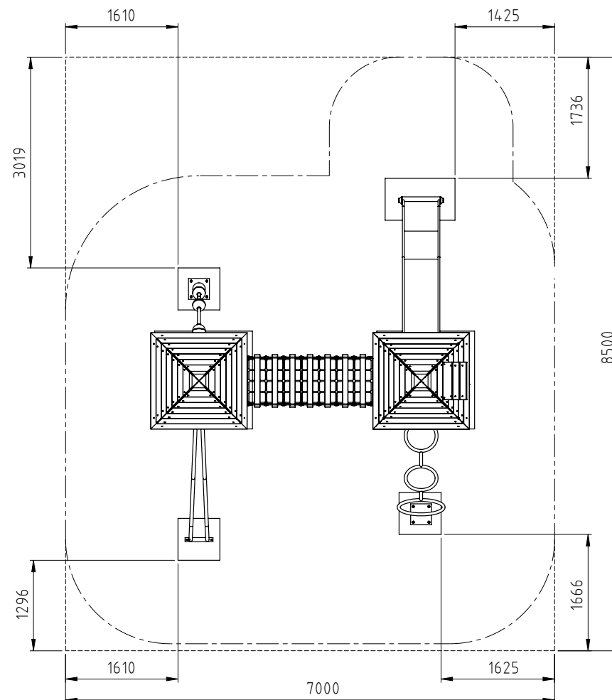
Skizze 3a: Draufsicht mit Fundamentlage
