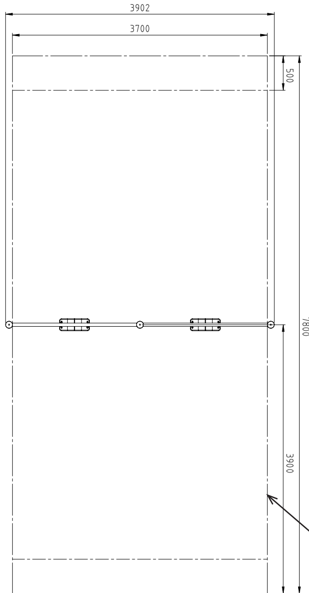
Skizze 4: Draufsicht
