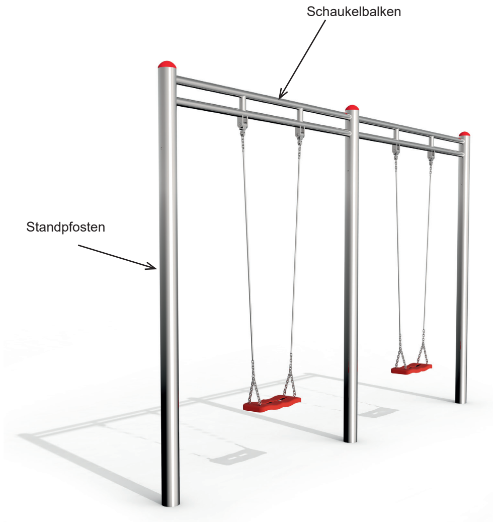
Skizze 1: Gesamtansicht des Spielgerätes
