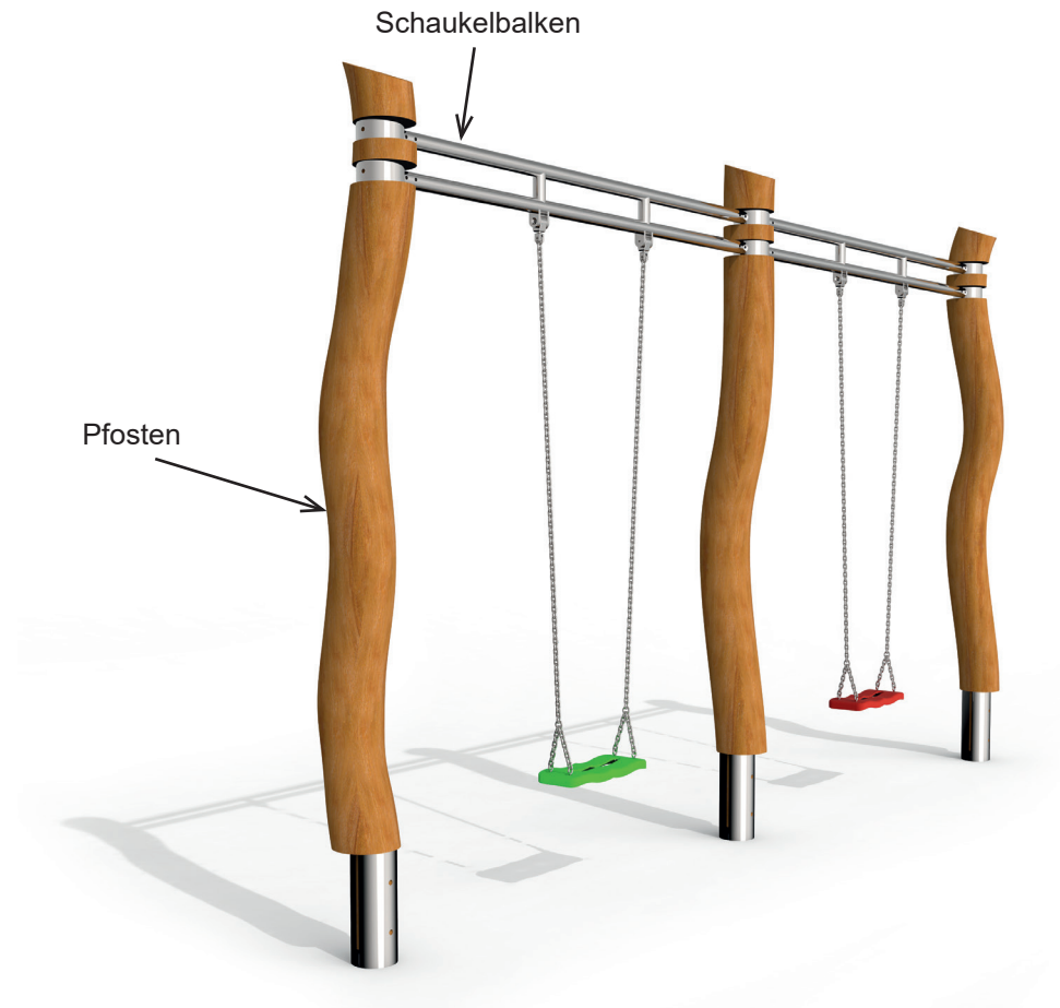
Skizze 1: Gesamtansicht des Spielgerätes
