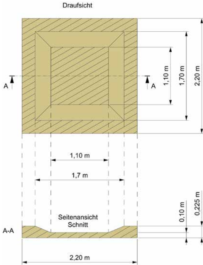
Skizze 2: Sickerschicht aus KFT-Material
