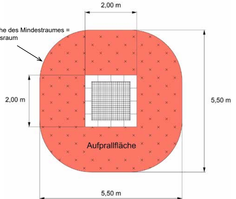
Skizze 4: Draufsicht
