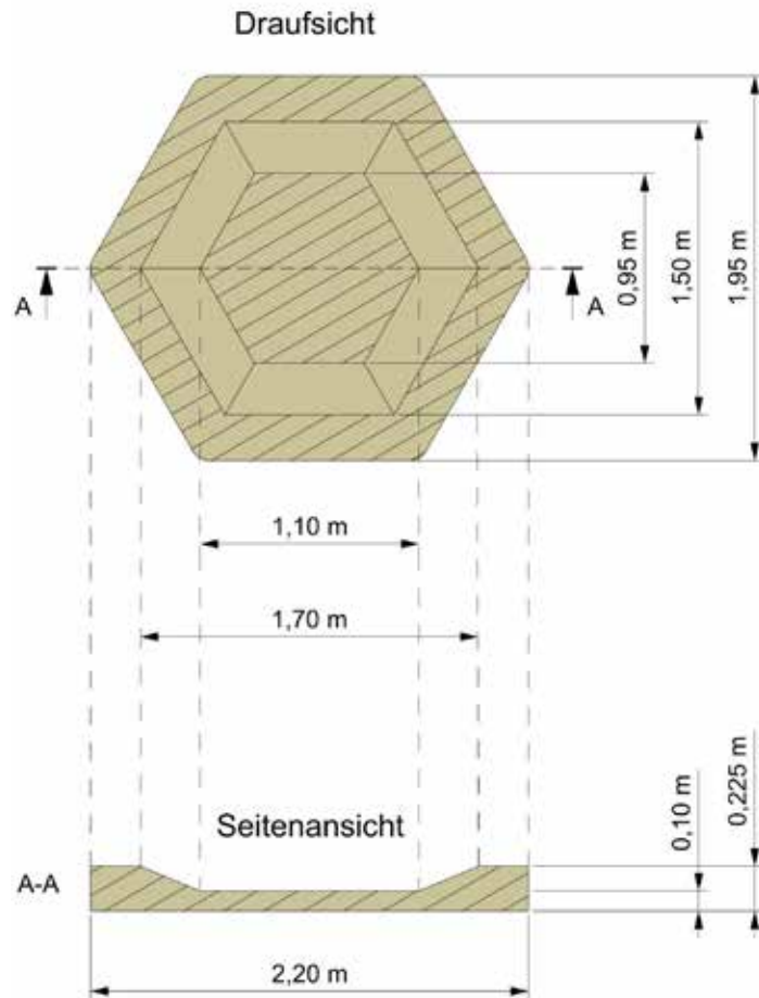
Skizze 2: Sickerschicht aus KFT-Material
