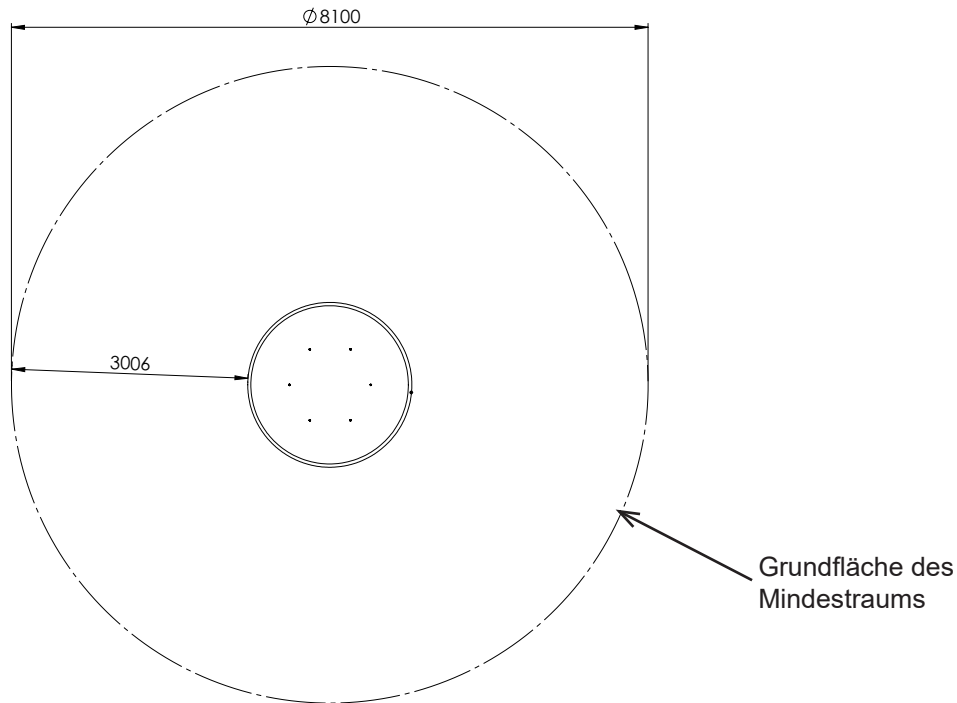
Skizze 3: Draufsicht
