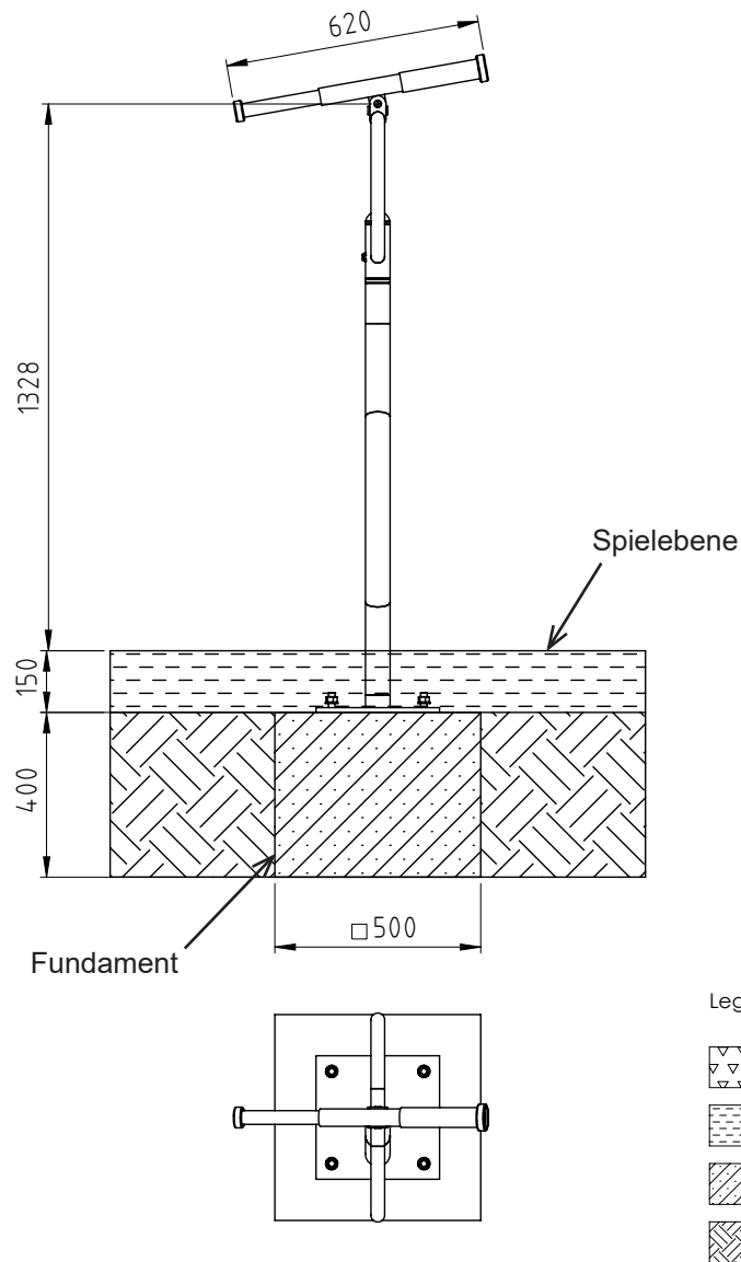
Skizze 2: Fundamentplan
