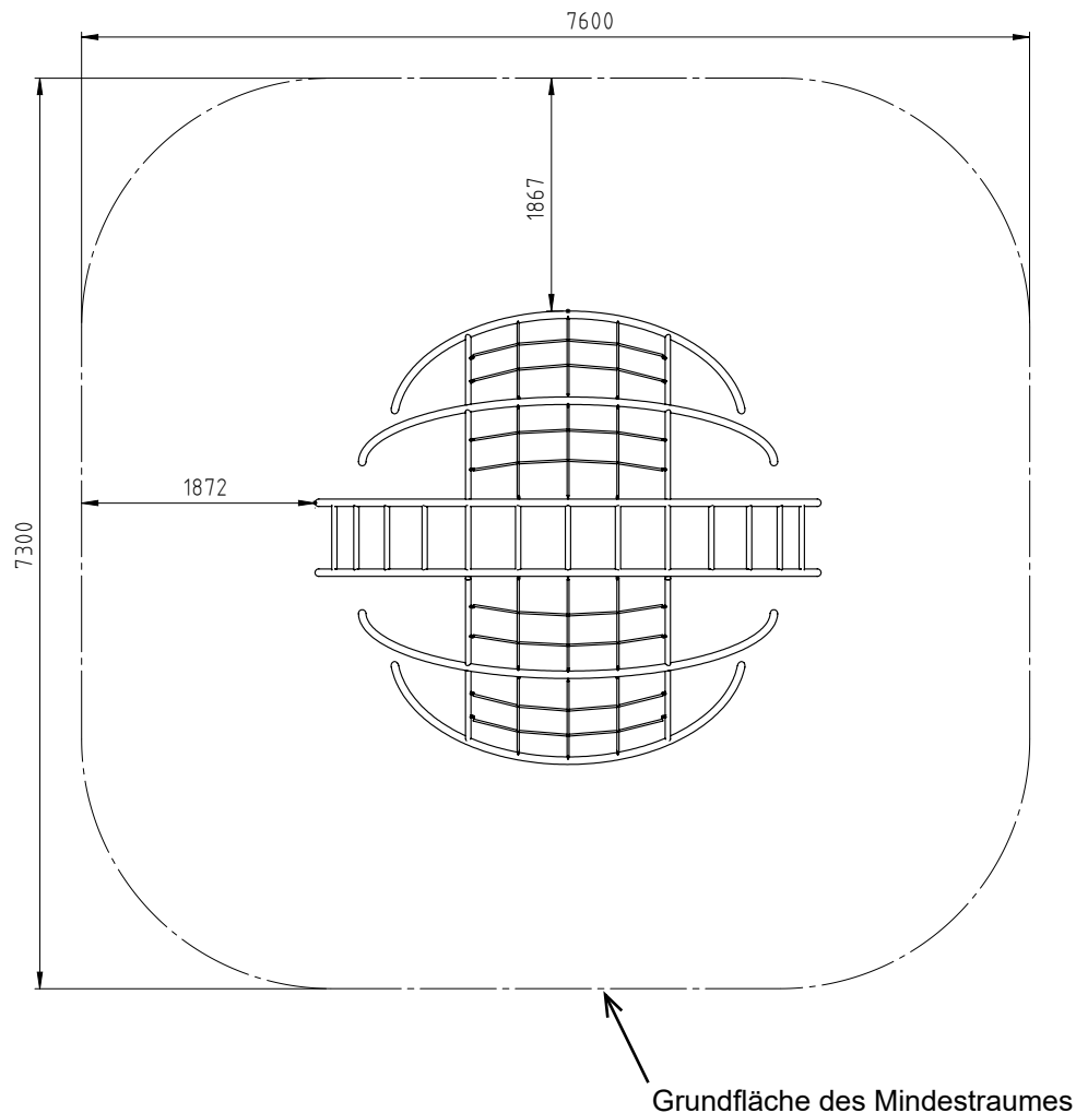
Skizze 4: Draufsicht
