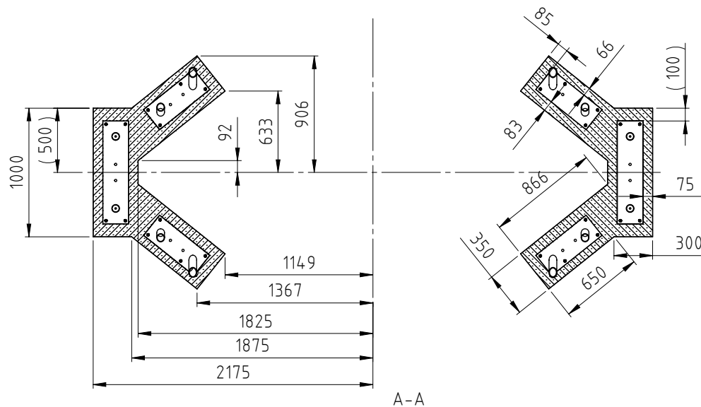
Skizze 3: Detailansicht Fundamentplan
