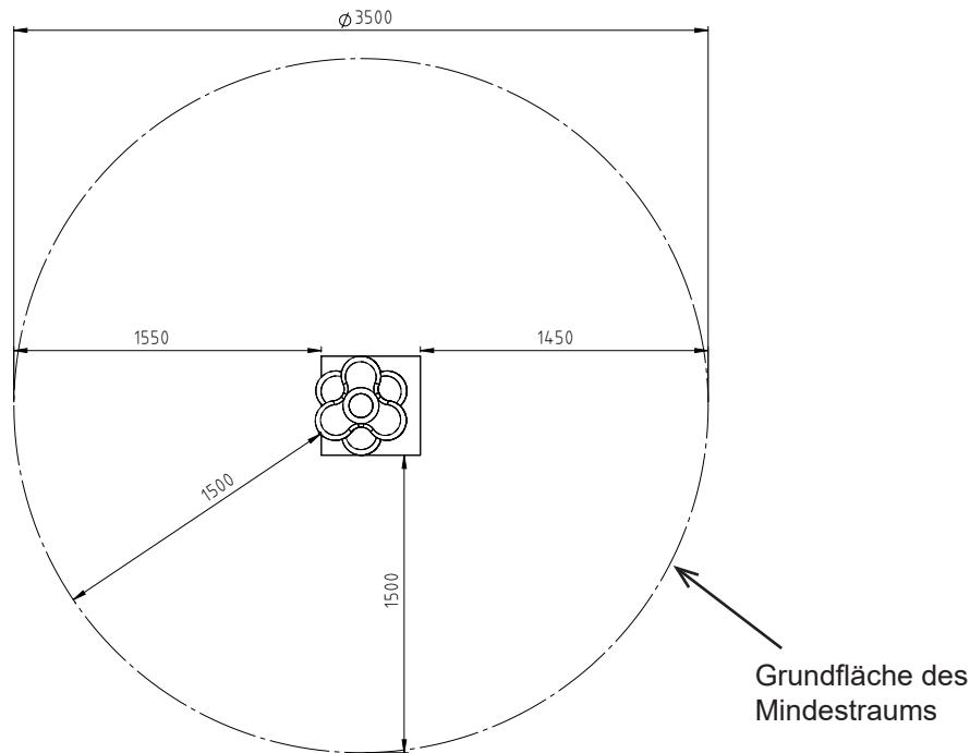
Skizze 3: Draufsicht
