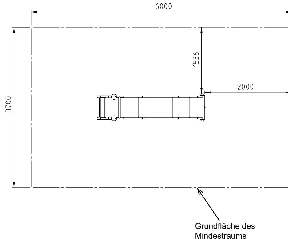
Skizze 3: Draufsicht
