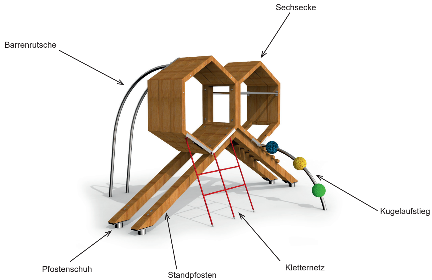
Skizze 1: Gesamtansicht des Spielgerätes
