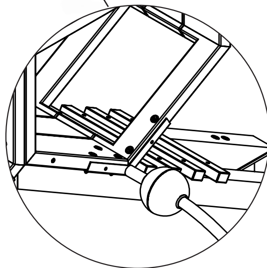
Skizze 4b: Anbindung Kugelaufstieg, Barrenrutsche
