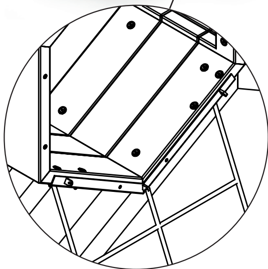
Skizze 4a: Anbindung Kletternetz
