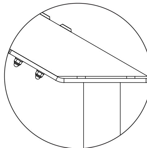
Skizze 4c: Anbindung Pfostenschuh
