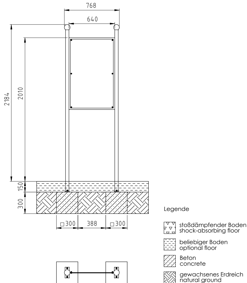
Skizze 4: Fundamentplan Instruktionsstafel
