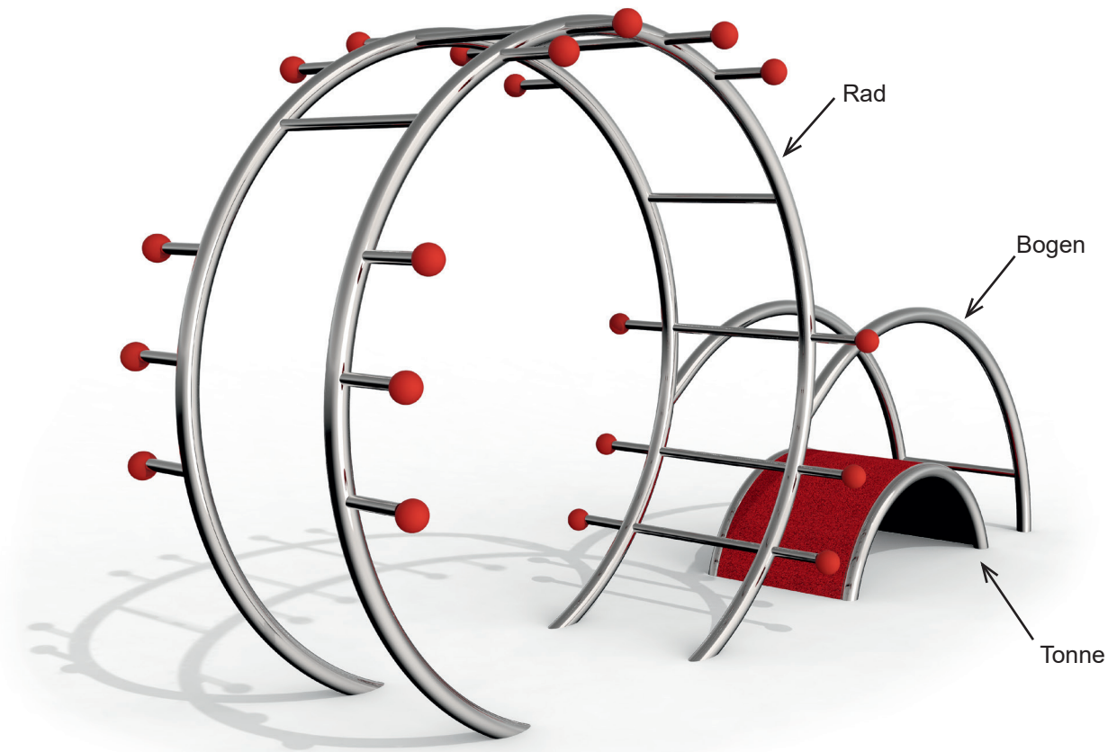
Skizze 1: Gesamtansicht des Fitnessgerätes
