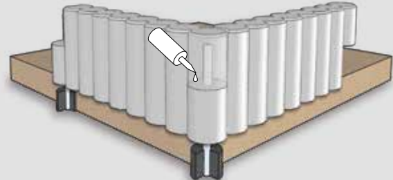
Einfundamentierung des Kettenelements mit Hilfe von verlängerten Montagerohren auf losem Untergrund. Eine Verklebung der Elemente untereinander ist erforderlich.
