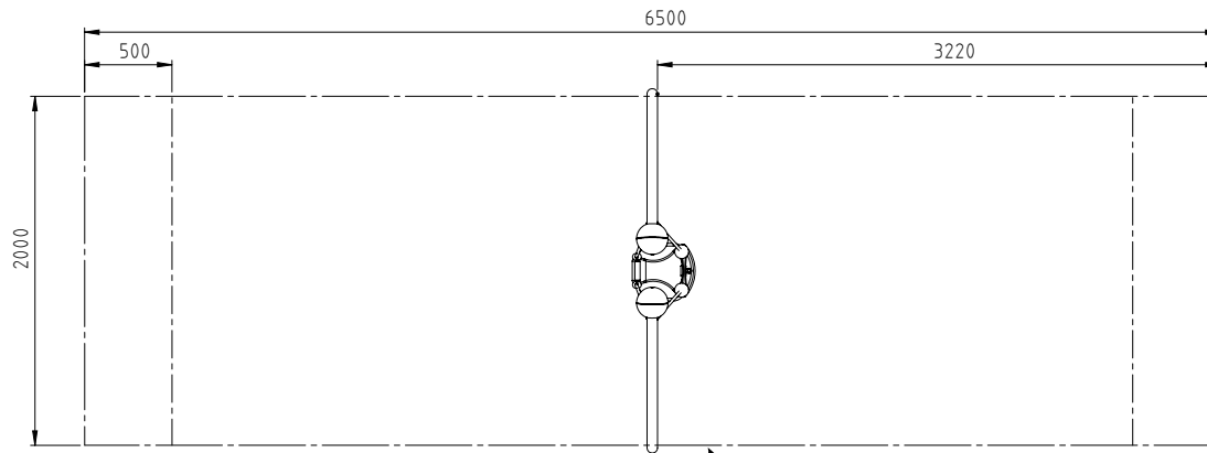
Skizze 3: Draufsicht
