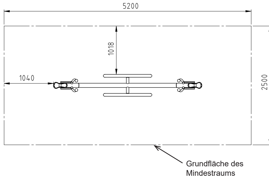
Skizze 3: Draufsicht
